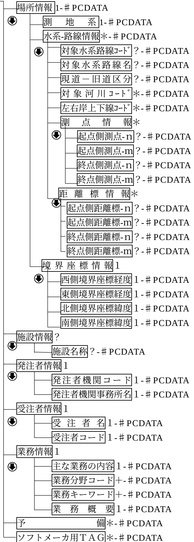
図付 1-1 業務管理ファイルの DTD の構造
